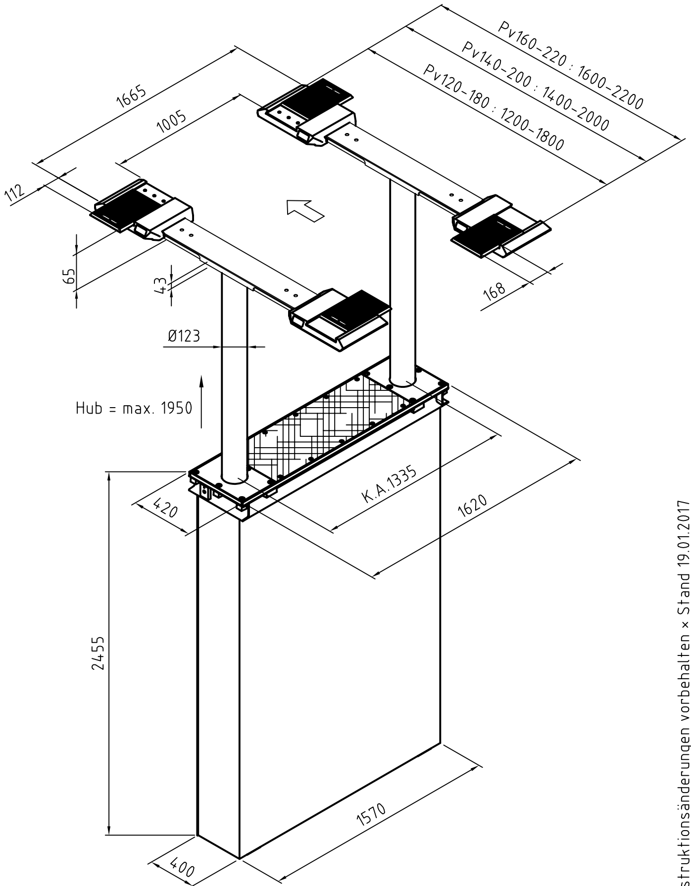
Maßskizze incl. Angabe der Überfahrhöhen
