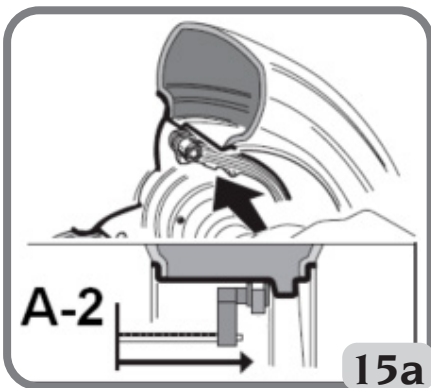
Zentrum der Aussparung des Halters ohne Gewichte
