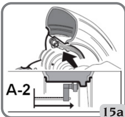
Centre de l'encoche de l'outil sans porte-masse
