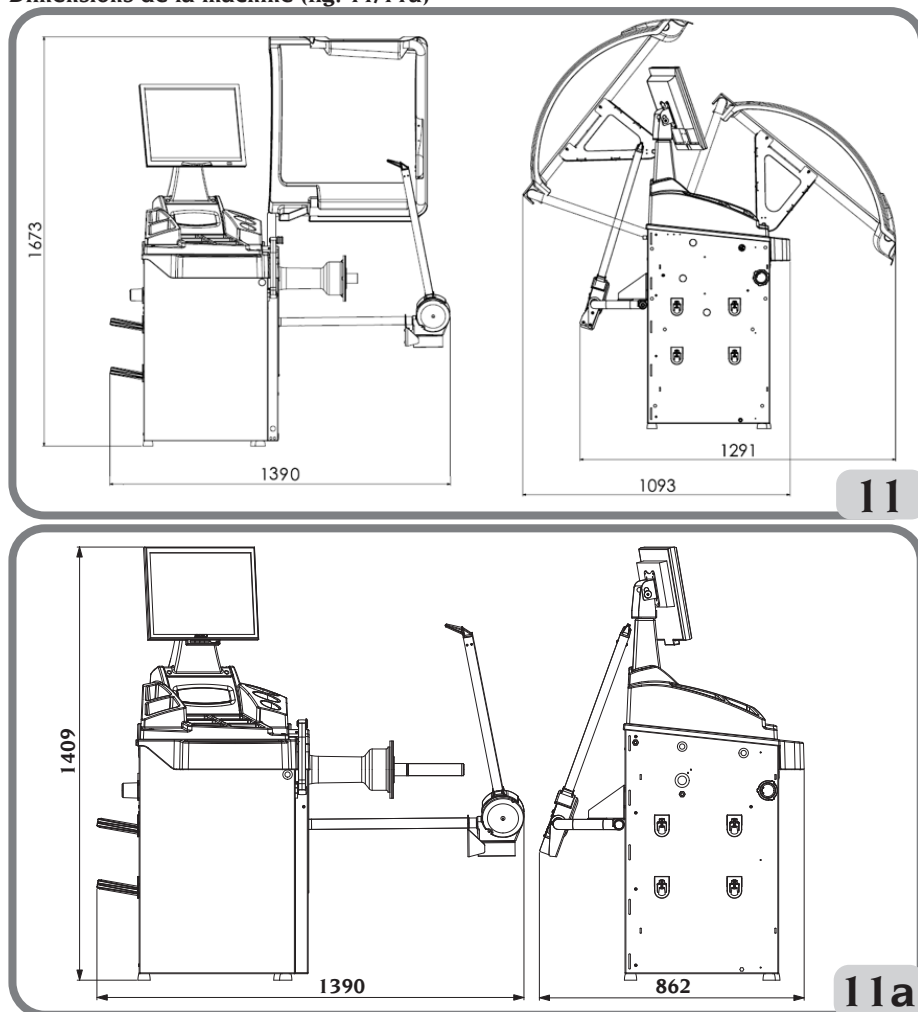
Dimensions de la machine (fig. 11/11a)
