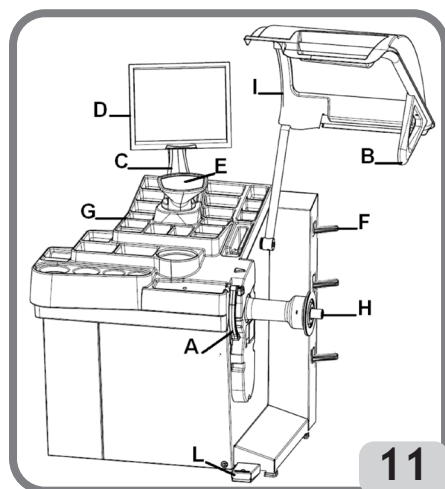
Principali elementi di funzionamento (fig. 11)
