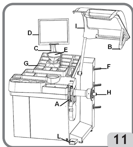
Éléments principaux de fonctionnement (fig. 11)
