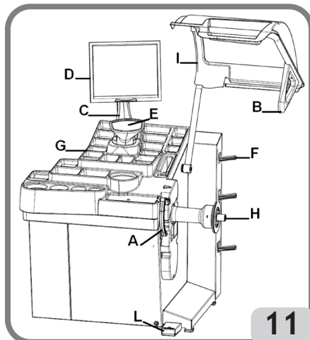
A) Automatischer Messarm für Durchmesser
