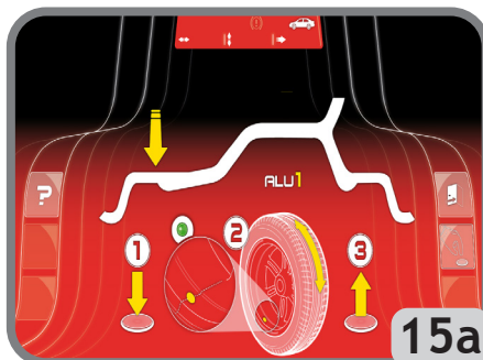
Position 2 masse adhésive
