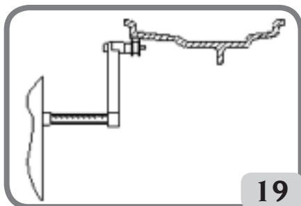
Fig.19 : Acquisition automatique de la distance et du diamètre du plan interne dans le Type de Programme ALU 1P
