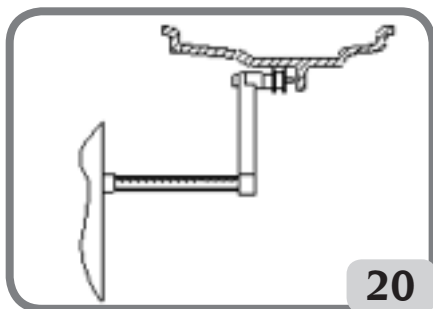
Fig.20: Acquisizione automatica della distanza e del diametro del piano esterno nel Tipo di Programma ALU 1P e ALU 2P
